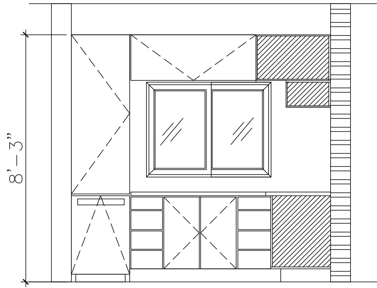
KITCHEN ELEV DET 7 SCALE: 1/2" = 1"
